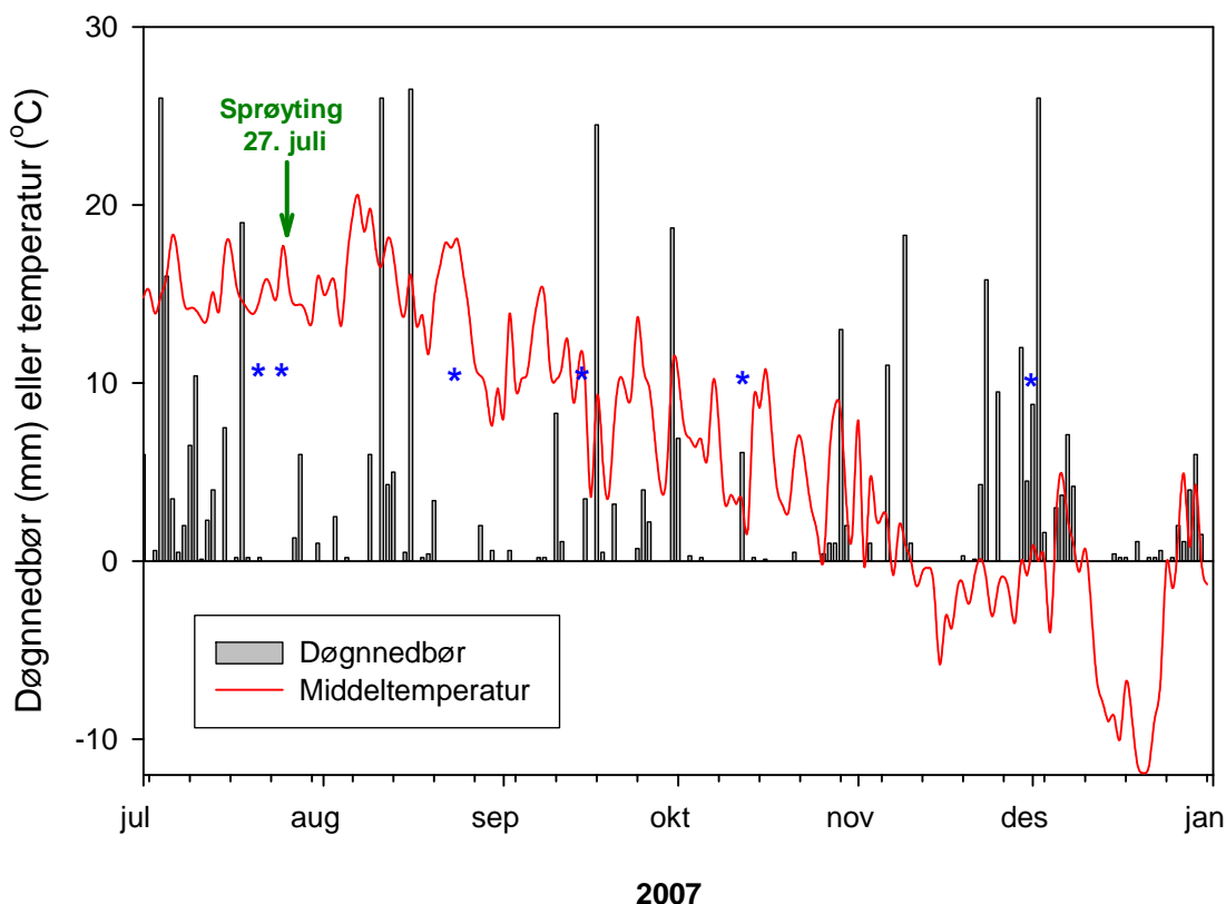
Figur 13. Døggnedbør (mm) og døgnmiddeltemperatur (°C) på Gardermoen, klimastasjon 478, i perioden juli-desember 2007. Tidspunkt for vannprøveuttak er markert med blå stjerner.
