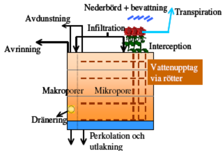
Figur 12. Modellstruktur for simuleringsmodellen MACRO.
