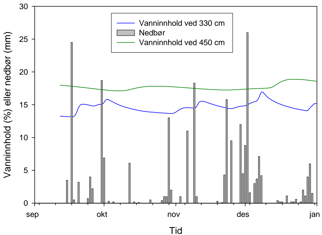
Figur 15. Gjennomsnittlig vanninnhold (%) ved to jorddyb (330 cm og 450 cm) sammenlignet mot døgnedbør (mm) fra 12. september 2007 til 1. januar 2008.
