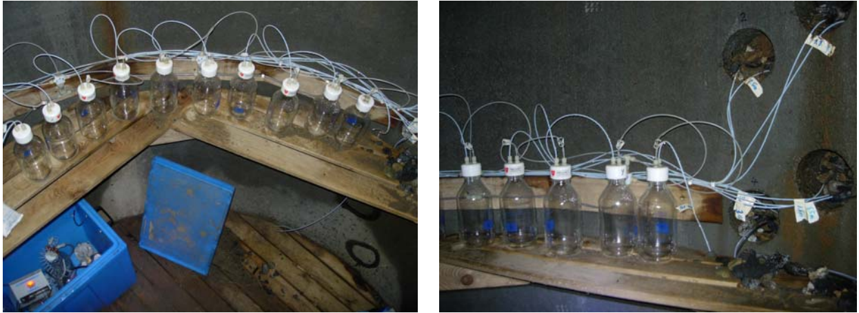
Figur 5. Sondene i jorda og vannprøveflaskene i lysimeterkummen er forbundet med teflonslanger. Glassflaskene er koblet i serie og står under konstant sug ved hjelp av en 12 V vakuumpumpe med vakuumregulator (i blå boks). Foto: Marit Almvik.
