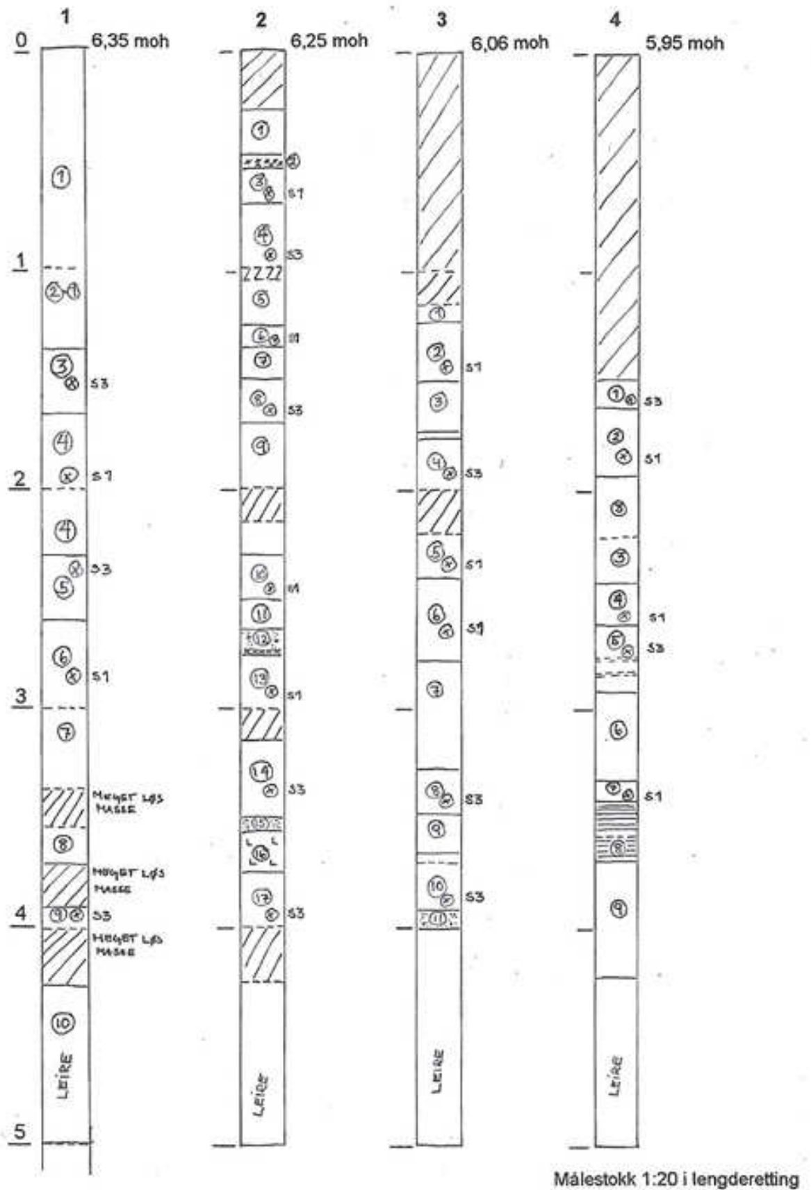
Figur 6A Tegning av boresøylar 1 til 4 fra område 1. Diagonal skraving markerer forstyrret masse. Horizontal tett skraving markerer tett, kompakt treverk. Prikker markerer sand.
