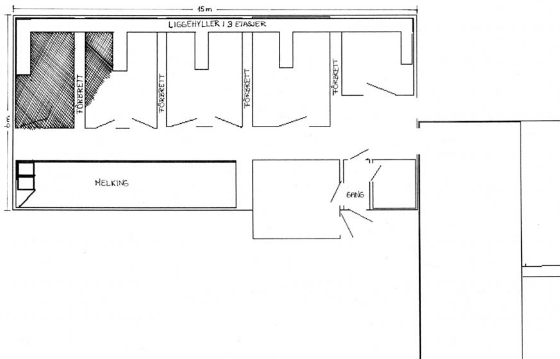
Figur 3. Skisse av geitefjøset på Aalan gard. Liggehyller i tre etasjar. Teikning: Knut Åland og Heidi Nilssen.
