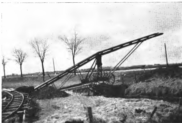
Fig. 4. Fra Tetenhusen, Schleswig-Holstein. Transportør for lessing av maskintorv m. v.
