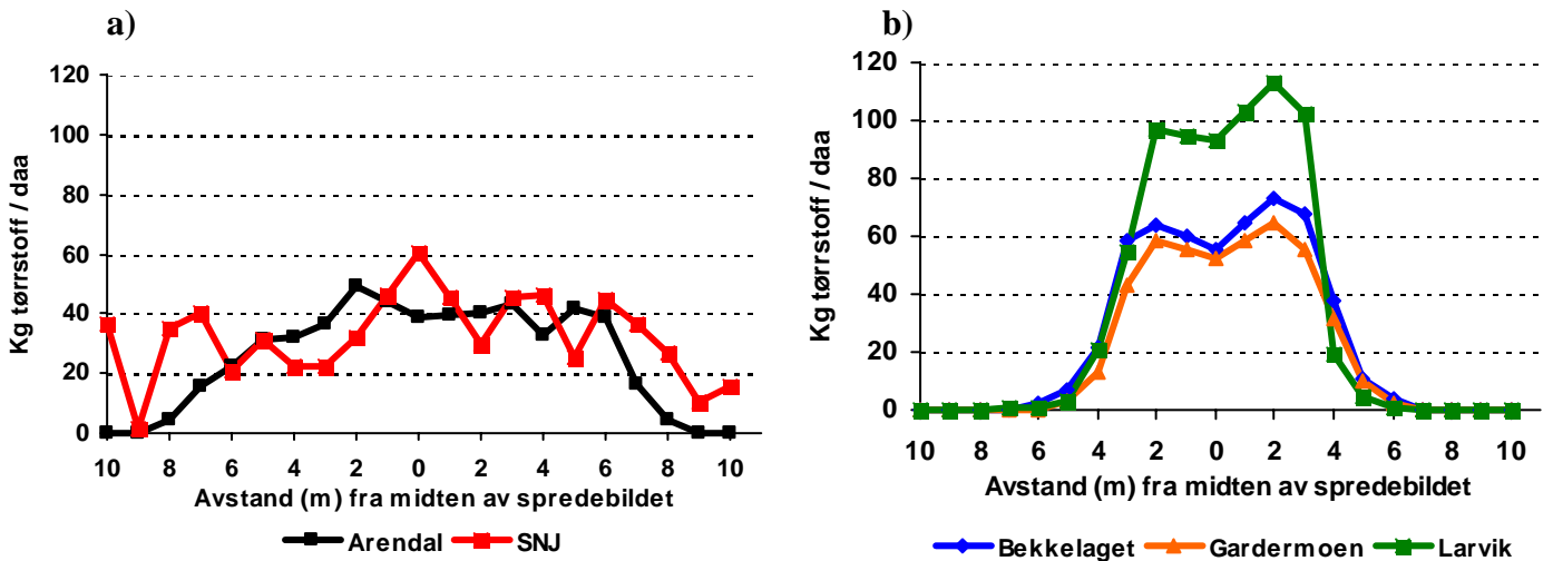
Figur 12. Spreddebildet ved spredning av slampellets (a) og slamgranuler (b) ved kjøring med pendelspreder (Vicon) ved full utmatingsåpning.
