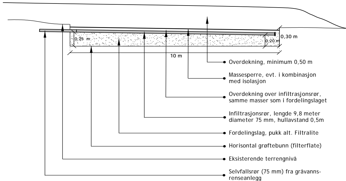
Prinsippkisse av grunn etterpuleringsgrøft for infiltrasjon av rensset vann fra gråvannfilteranlegg
