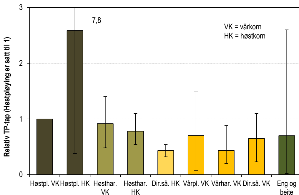
Figur 3.2 Gjennomsnittlig effekt av ulike typer jordarbeiding i nordiske ruteforsøk
