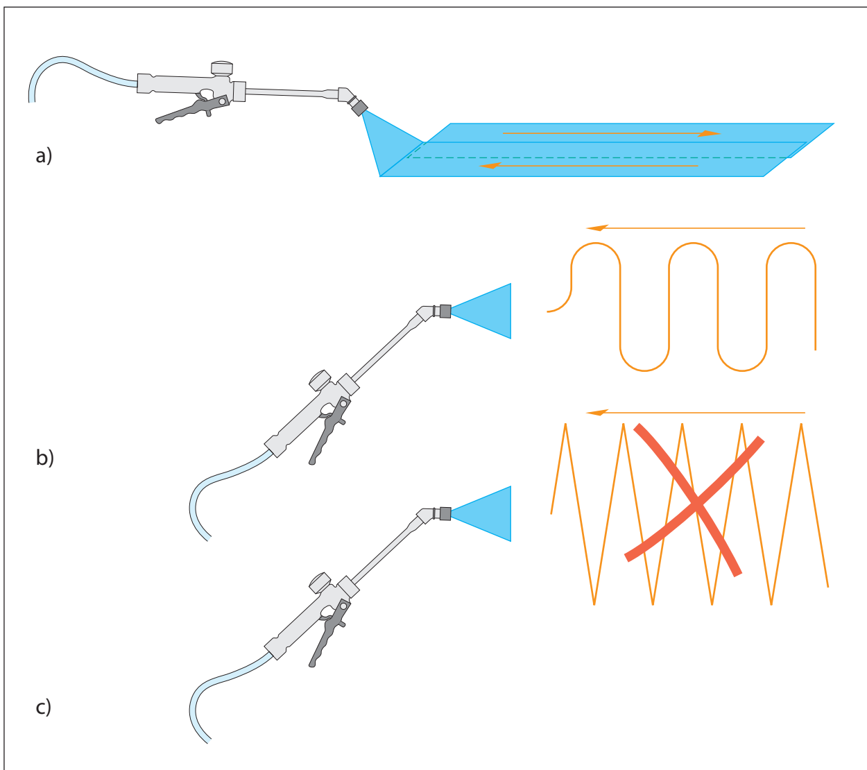
Figur 31. Jevne, rette 50 % overlappende drag gir best sprøyteresultat (a), sprøyt i avrundede bevegelser og med jevn dyseføring (b) og unngå siksakk bevegelser med ujevnt overlegg og ujevn hastighet (c). Illustrasjon: Bjørn Norheim.
