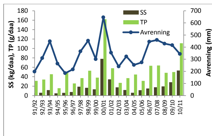
Figur 11. Avrenning og tap av totalfosfor (TP) og suspendert stoff fra 1991 til 2011 beregnet for jordbruksarealet.
