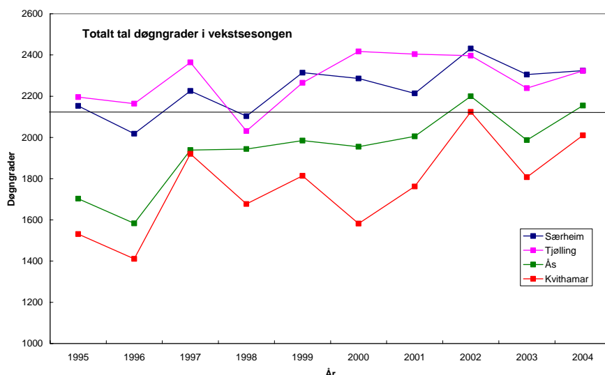
Figur 1. Akkumulerte døgngader (basetemperatur 0 °C) i utrekna vekstsesong på fire lokalitetar i 10 år. Det er trekt ei line gjennom verdien for Kvithamar i 2002.
