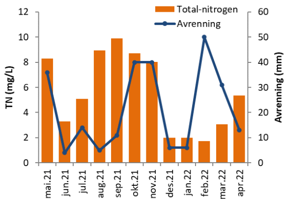
Figur 6. Avrenning og vannføringsveide konsentrasjoner av totalnitrogen (TN) i 2021/2022.
