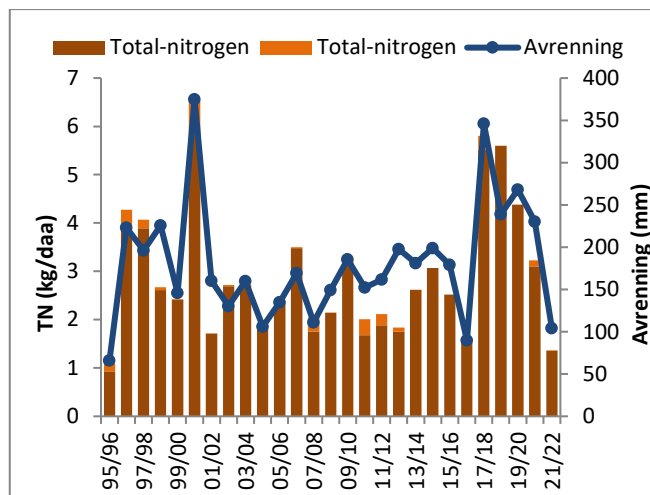
Figur 7. Tap av totalnitrogen i grøft og på overflate i perioden fra 1995/1996 til 2021/2022.
