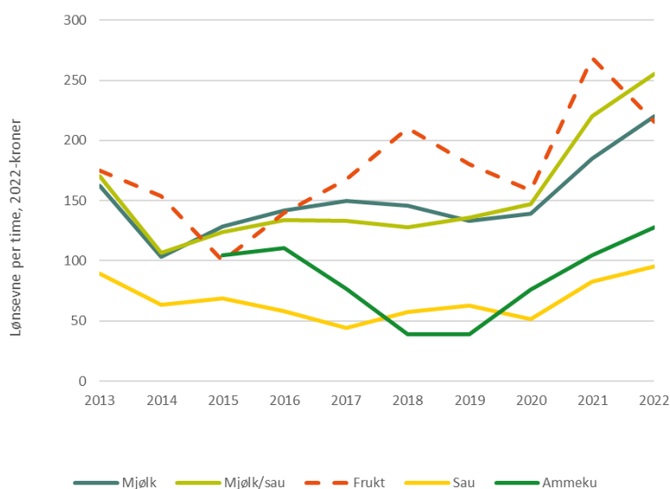
Figur 3-7 Lønsevne per time for ulike driftsformer på Vestlandet.
